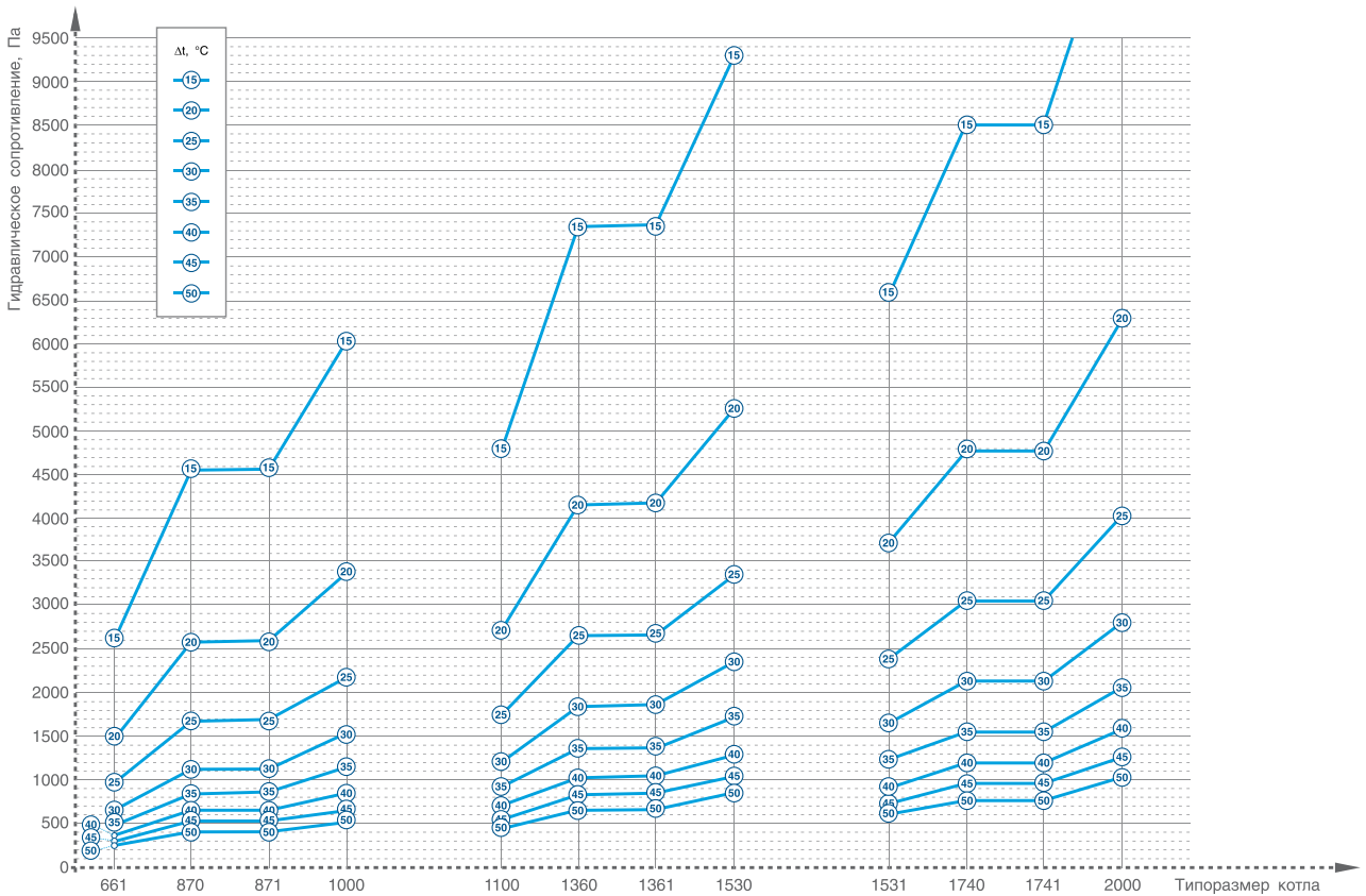
Зависимость гидравлического сопротивления котлов ТТ50 от Δt. Продолжение
