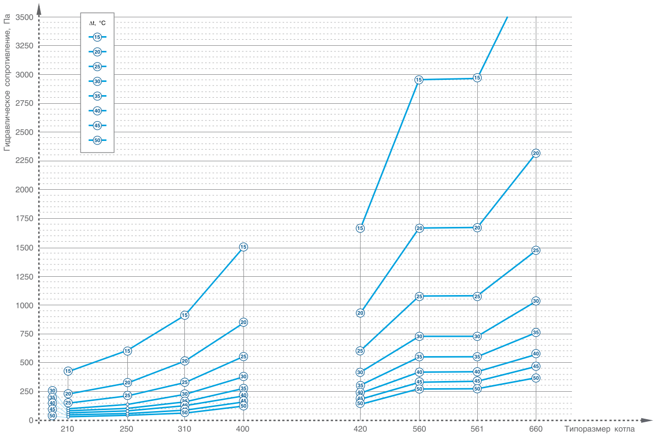
Зависимость гидравлического сопротивления котлов ТТ50 от Δt
